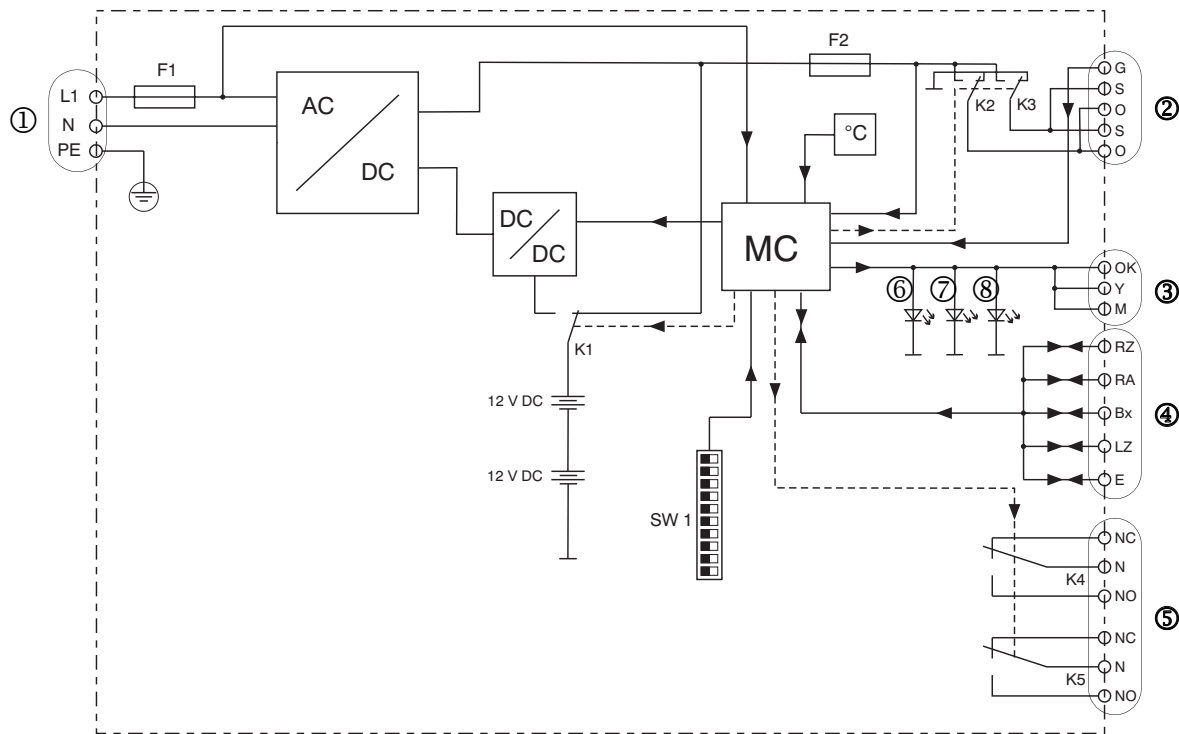
Abbildung 3: Blockschaltbild
