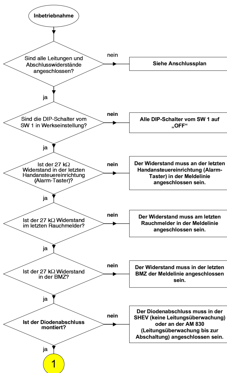
Abbildung 13: Inbetriebnahme – Checkliste
