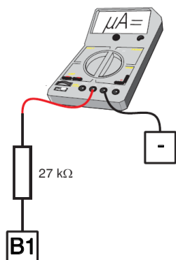
Abbildung 23: Schleifenstrom Hauptbedienstellenanschluss „B1“
