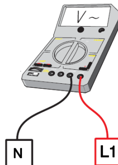
Abbildung 16: Spannung Netz
