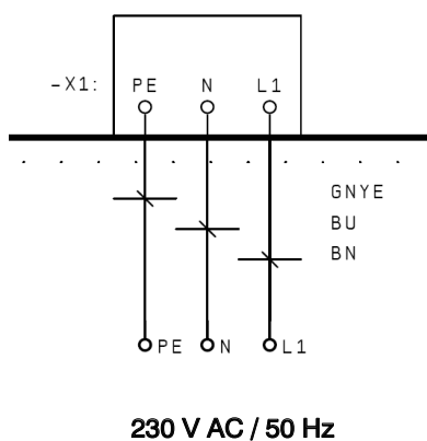
Abbildung 6: Anschlussplan Netz
