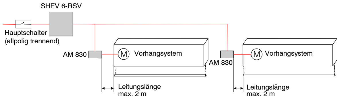
Abbildung 10: Anschlussschema Einzelroller über zentrale Energieversorgung
