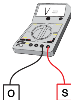
Abbildung 17: Spannung Motoranschluss
