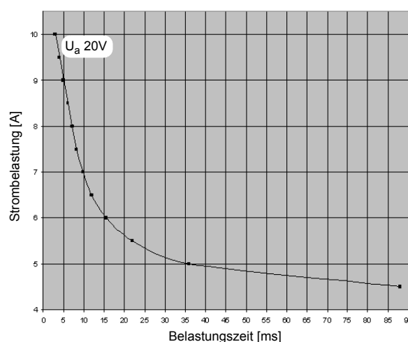
Abbildung 1: Diagramm Ausgangs-Impulsbelastung
