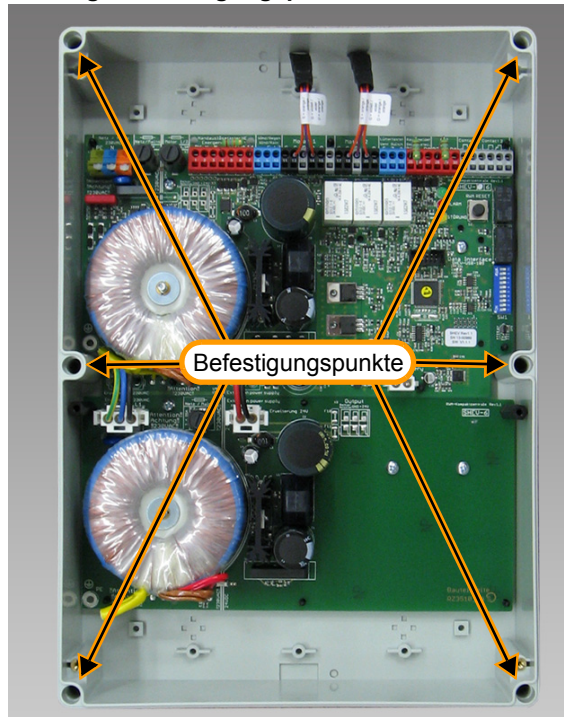
Abbildung 4: Befestigungspunkte Gehäuse
