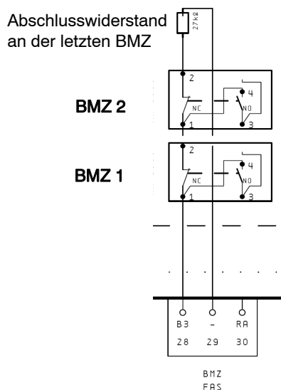
Abbildung 12: Anschlussplan Kontakt BMZ
