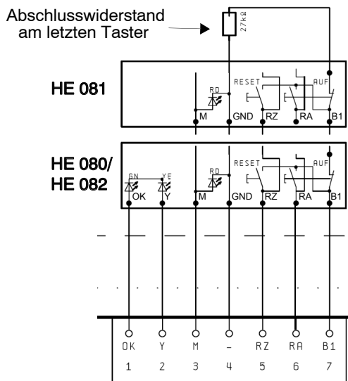
Abbildung 8: Anschlussplan Handansteuereinrichtung (Alarm-Taster)
