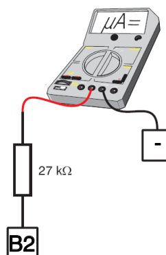
Abbildung 25: Schleifenstrom Rauchmelderanschluss
