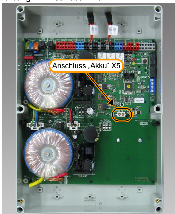
Abbildung 14: Anschluss Akku
