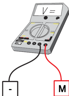
Abbildung 21: Spannung Hauptbedienstellenanschluss „M“ (Alarm)
