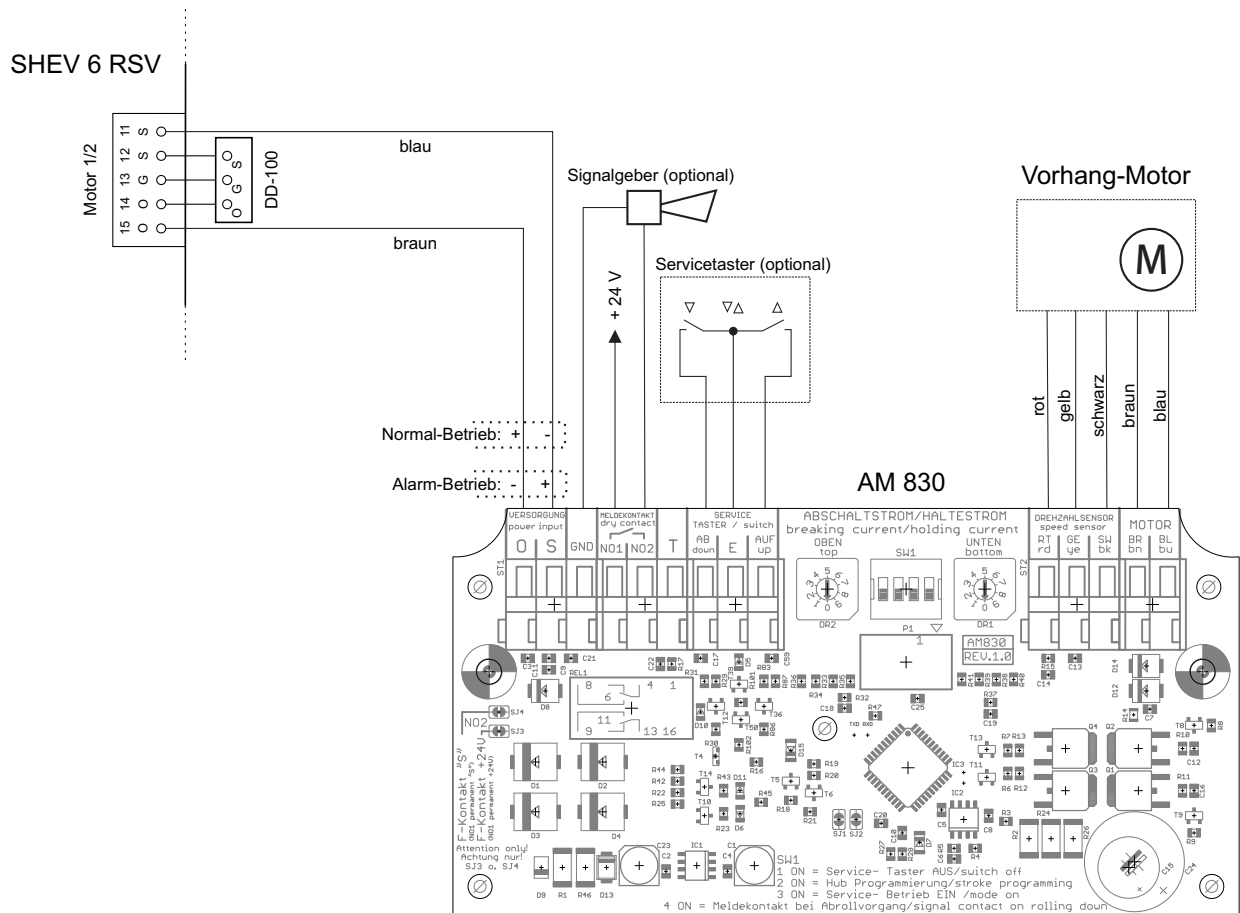
Abbildung 10: Anschlussschema Einzelroller über zentrale Energieversorgung
