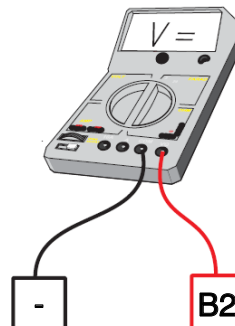
Abbildung 24: Spannung Rauchmelderanschluss
